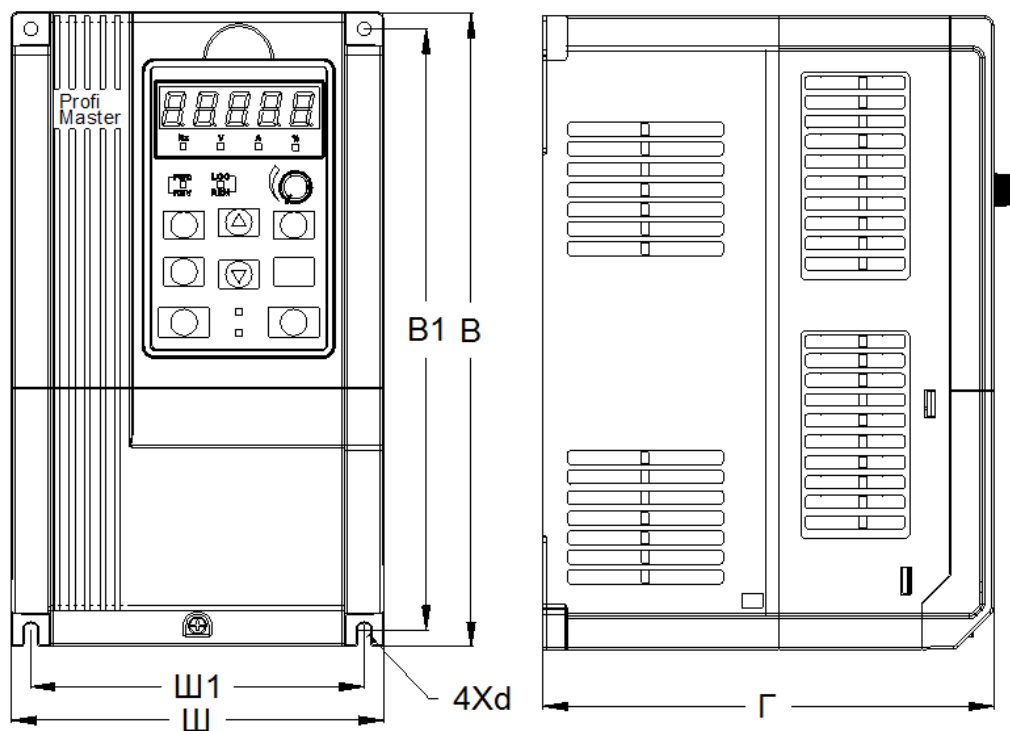
Рис. 2-7. ПЧ 4 – 22 кВт
