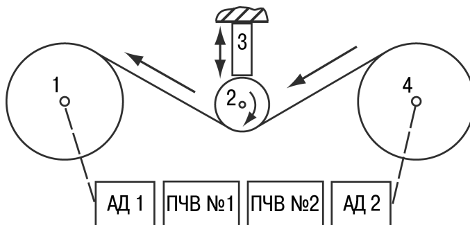
Рисунок 2.8 - Кинематическая схема перемоточного механизма
