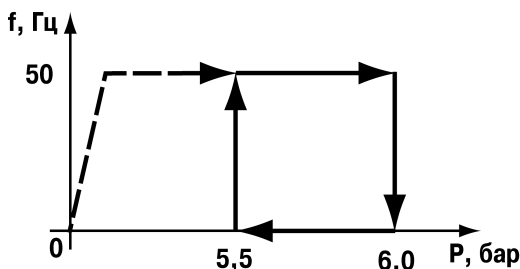
Рисунок 2.5 - Диаграмма релейного режима работы
