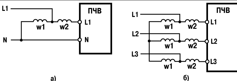
Рисунок 3.6 - Схема подключения питания к ПЧВ: с однофазным (а) и трехфазным (б) входом
