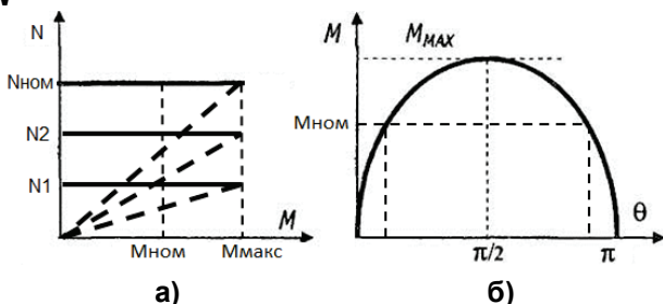
Рисунок 3.3 - Механические характеристики частотного регулирования СД (а) и распределение крутящего момента по полюсному делению (б)
