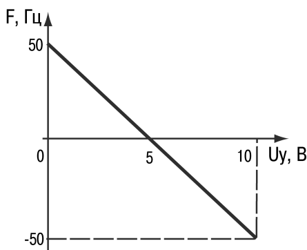
Рисунок 2.3 - Характеристика двунаправленного управления скоростью АД
