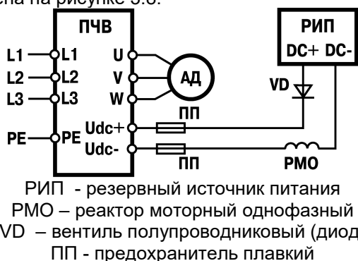
Рисунок 3.8 - Система основного/резервного питания ПЧВ
