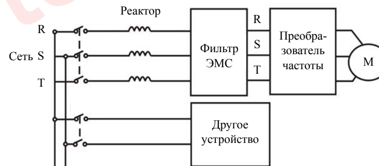
Рис. 4.14 Подключение входной цепи
