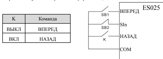
Рис. 6.14 Режим 3-проводного управления 1
