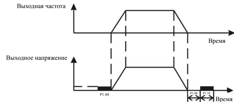
Рис. 6.5 График режима торможения постоянным током
