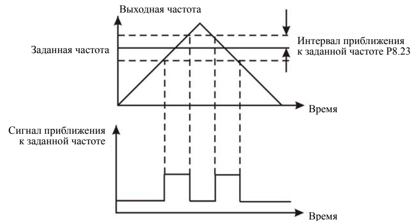
Рис. 6.23 Диаграмма сигнала приближения к заданной частоте
