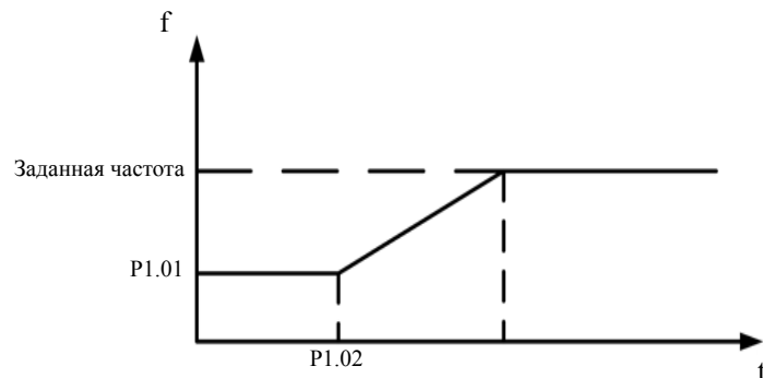
Рис. 6.4 Диаграмма запуска
