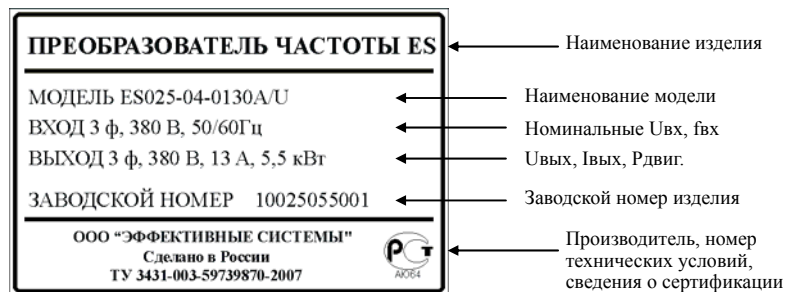
Рис. 1.2 Шильдик
